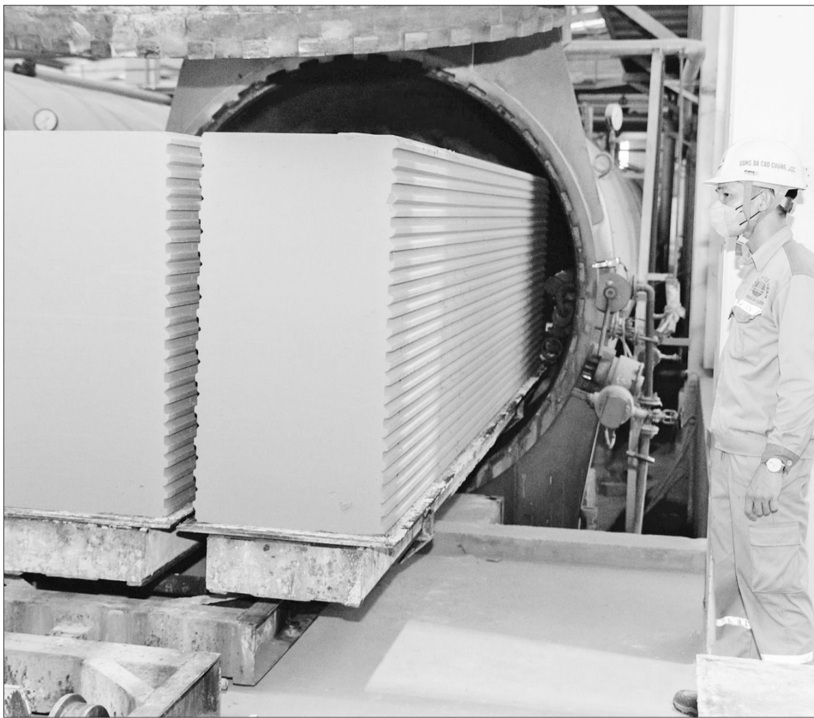
Sản xuất bê-tông chưng áp từ tro, xỉ tại nhà máy của Công ty cổ phần Sông Đà Cao Cường.
